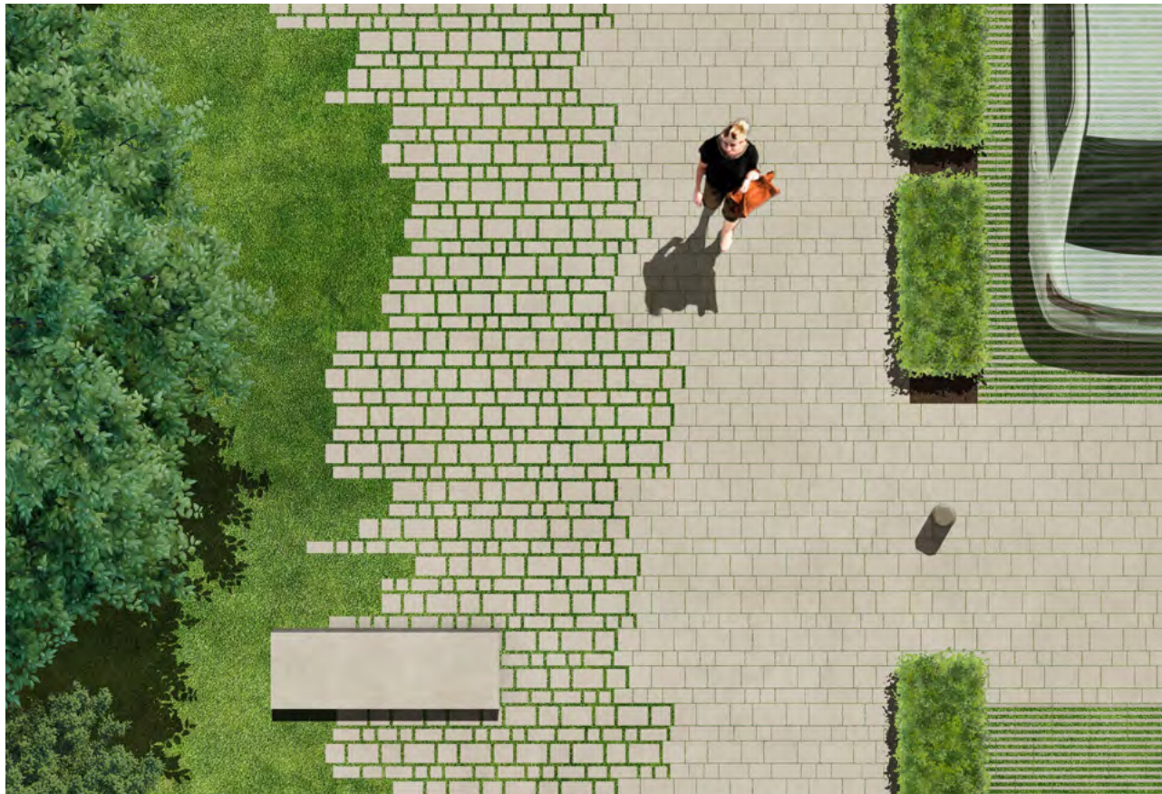
Schwammstadt Variante 5.1: Mehrsteinsystem Typ AB und Typ AB 30 mm gap, GDM.SCADA liner 5-5 40/40/12 cm, Reihenverband
